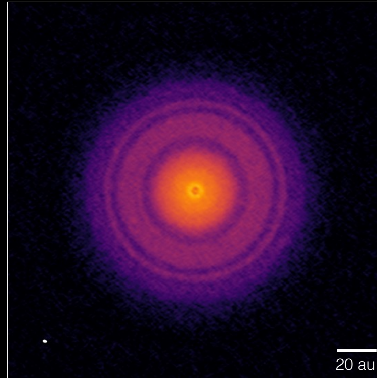
TW Hydrae
